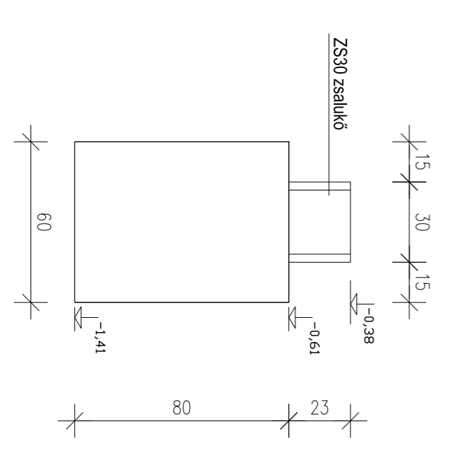
"A" KERESZTSZELVENY M=1:20 Készül 122,90 fm
